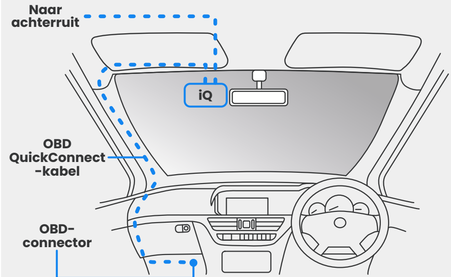
Geschatte plaatsing van de iQ-, OBD- en QuickConnect-kabel.
